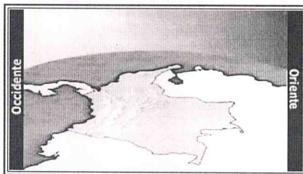
Posición actual aproximada del Sol respecto a Bogotá
